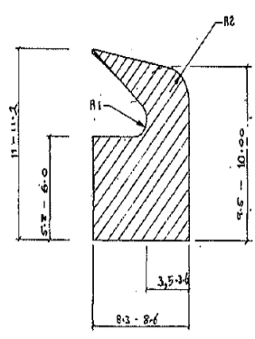
Die No: 377
