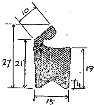
Die No: 938
