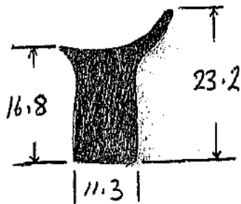
Die No: 589
