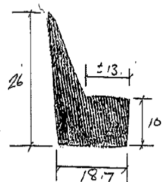
Die No: 899
