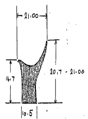
Die No: 414
