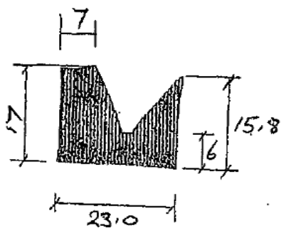
Die No: 719
