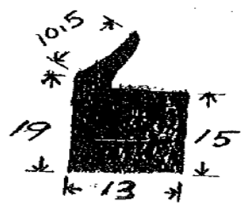
Die No: 387
