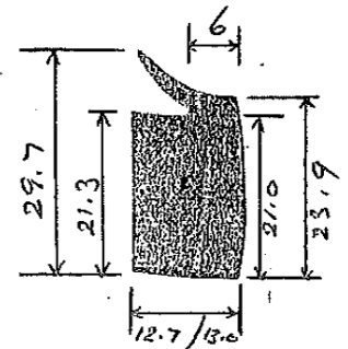
Die No: 657
