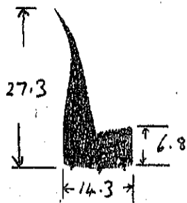
Die No: 571
