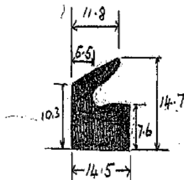
Die No: 615
