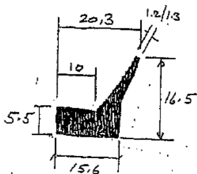
Die No: 841
