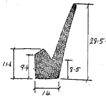
Die No: 898
