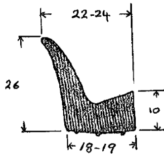
Die No: 447
