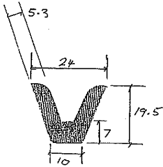
Die No: 919
