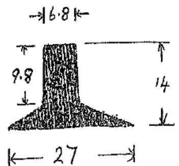
Die No: 632
