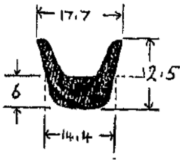
Die No: 544
