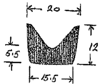
Die No: 590
