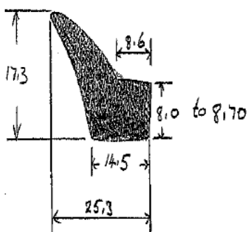
Die No: 614
