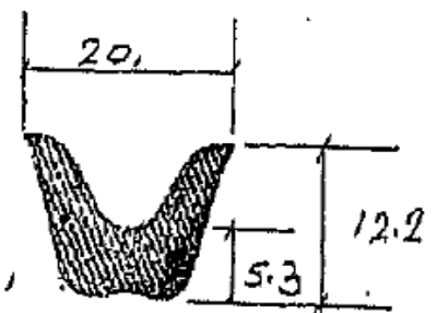
Die No: 716
