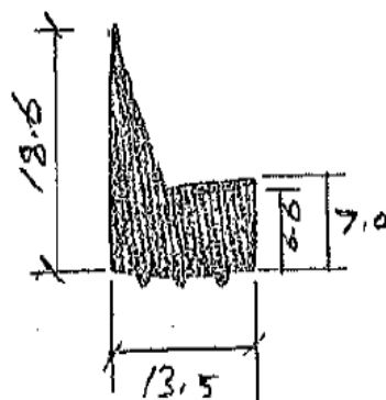
Die No: 898
