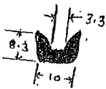
Die No: 328
