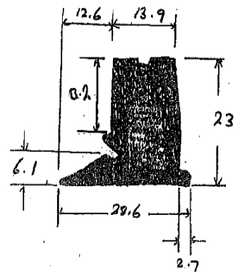
Die No: 632
