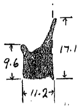
Die No: 387
